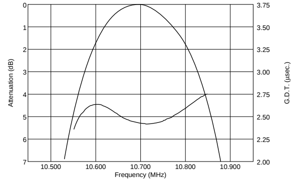
SFELA10M7GALP03-B0
