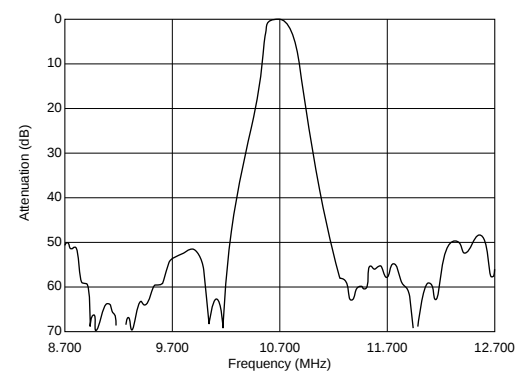
SFELA10M7GA0G-B0
