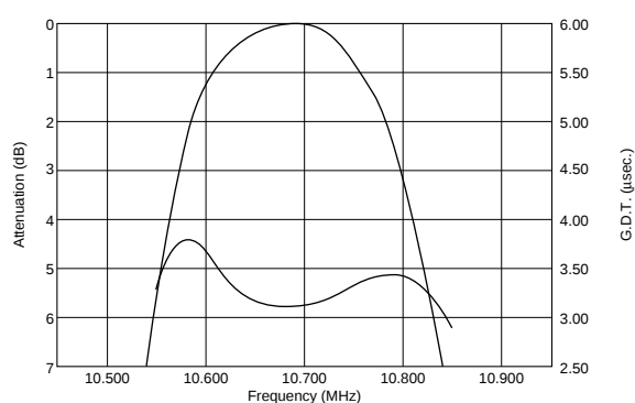
SFELA10M7GA0G-B0
