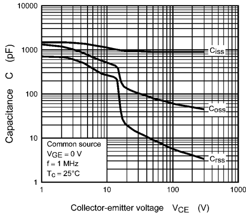
Fig. 8.13 C - V_{CE}
