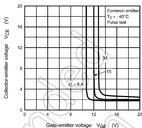
Fig. 8.2 V_{CE} - V_{GE}
