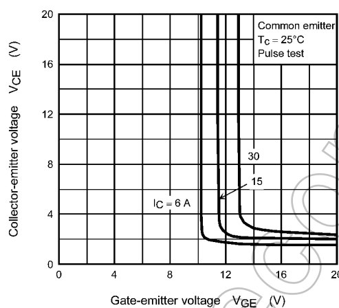
Fig. 8.3 V_{CE} - V_{GE}
