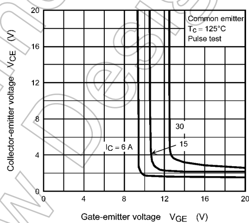
Fig. 8.4 V_{CE} - V_{GE}
