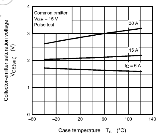
Fig. 8.6 V_{CE(sat)} - T_c
