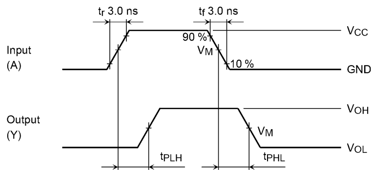
Fig. 9.8.1 t_{PLH} , t_{PHL}
