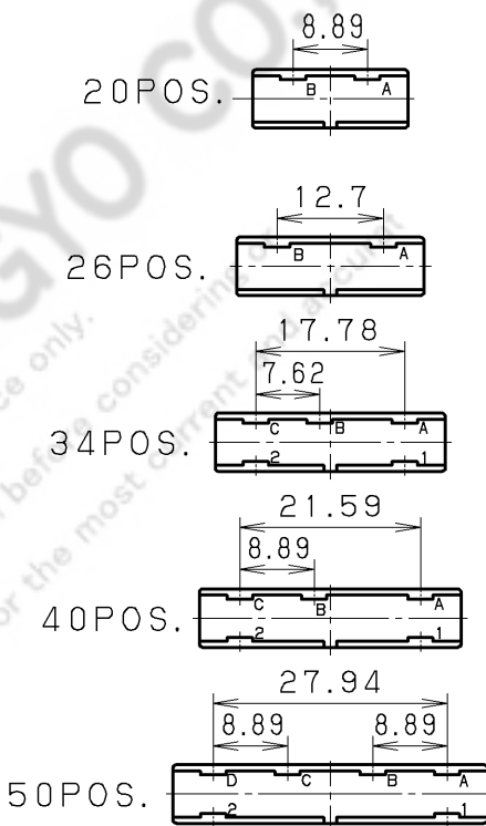
KEY POSITION DIM.
