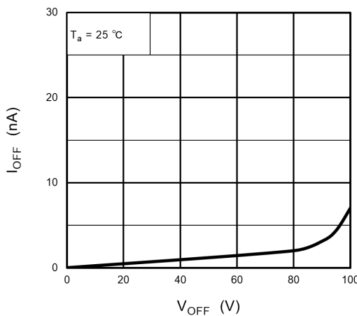
Fig. 12.10 I_{OFF} - V_{OFF}
