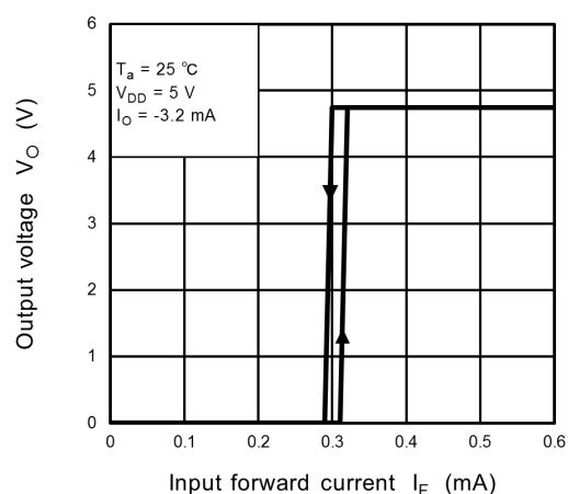
Fig. 12.2.10 I_F - V_O
