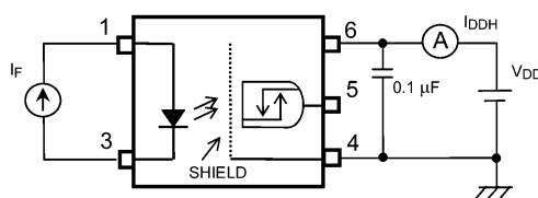
Fig. 12.1.4 I_{DDH} Test Circuit
