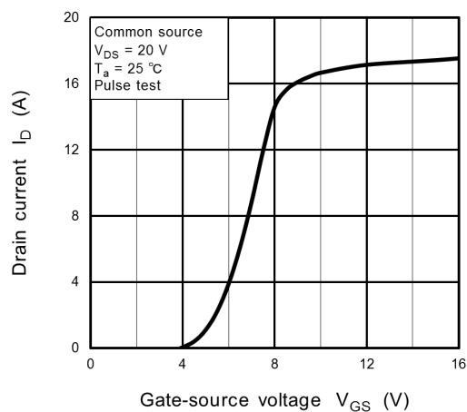
Fig. 8.3 I_D - V_{GS}
