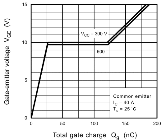
Fig. 8.7 V_{GE} - Q_g
