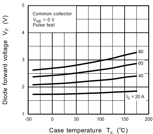
Fig. 8.12 V_F - T_c
