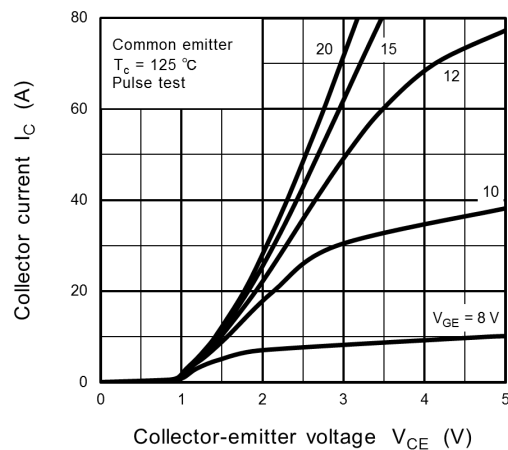
Fig. 8.3 I_C - V_{CE}
