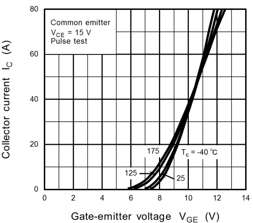
Fig. 8.6 I_C - V_{GE}
