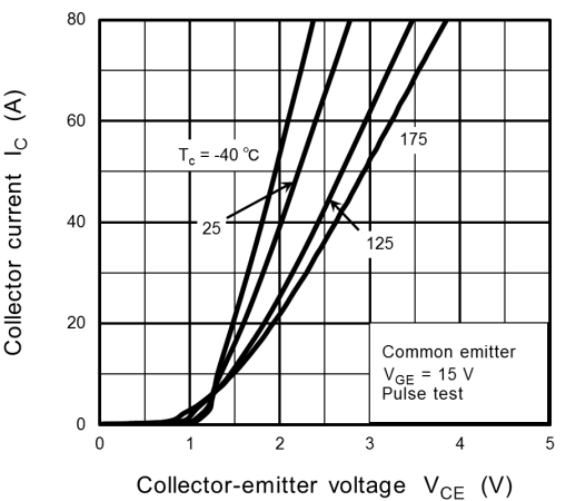
Fig. 8.4 I_C - V_{CE}
