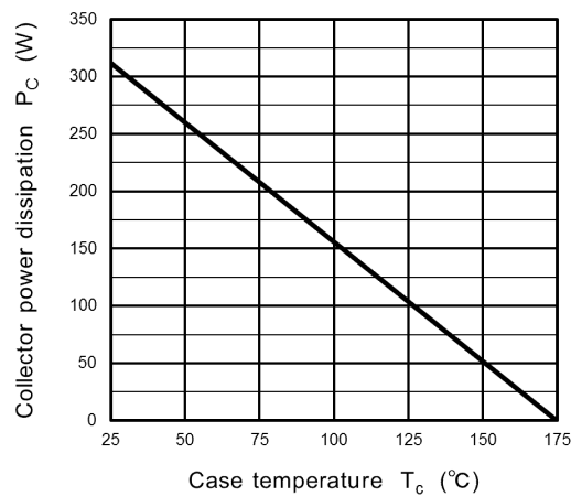
Fig. 8.13 P_C - T_c
