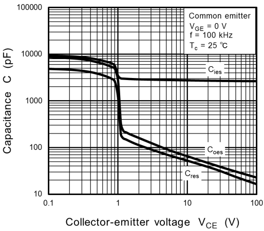
Fig. 8.8 C - V_{CE}
