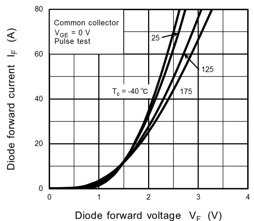
Fig. 8.11 I_F - V_F
