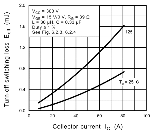
Fig. 8.15 E_{off} - I_C
