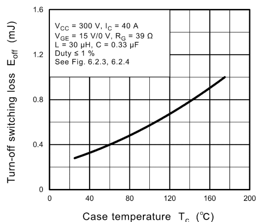
Fig. 8.17 E_{off} - T_c
