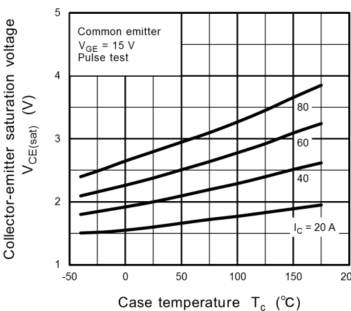
Fig. 8.5 V_{CE(sat)} - T_c
