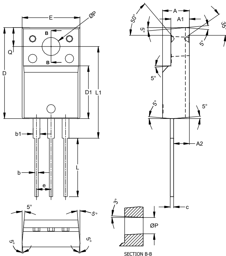
ITO220AB
