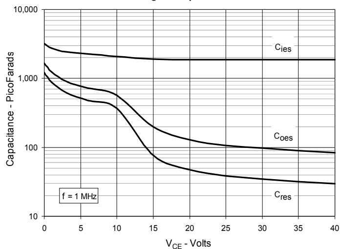
Fig. 9. Capacitance
