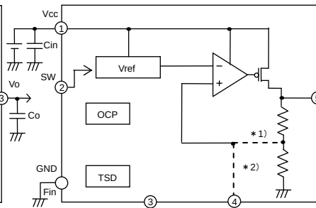
Fig.14 TO252-5
