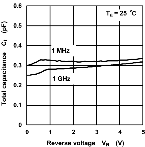
Fig. 9.3 C_t - V_R
