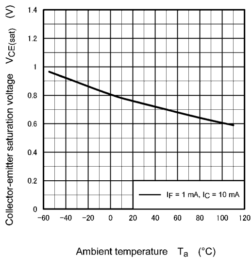
Fig. 11.11 VCE(sat) - Ta
