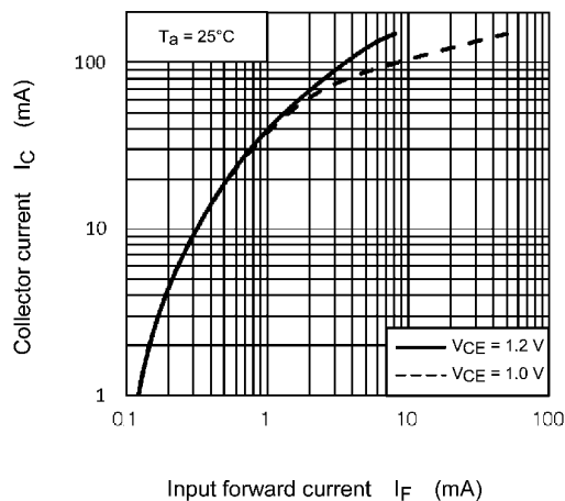
Fig. 11.8 IC - IF
