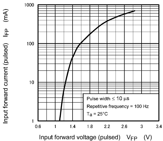
Fig. 11.6 I_{FP} - V_{FFP}
