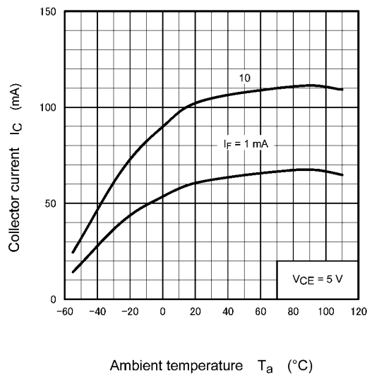
Fig. 11.12 IC - Ta
