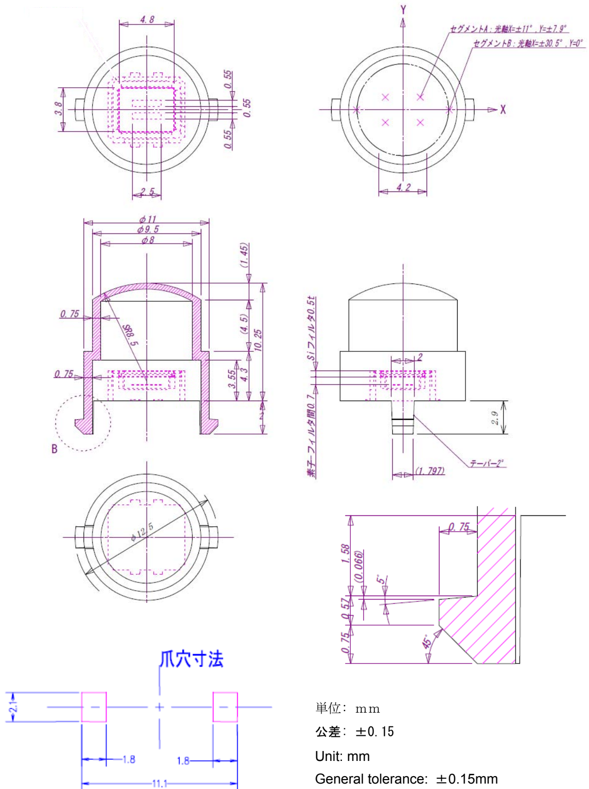
第 1 図 外形寸法図
