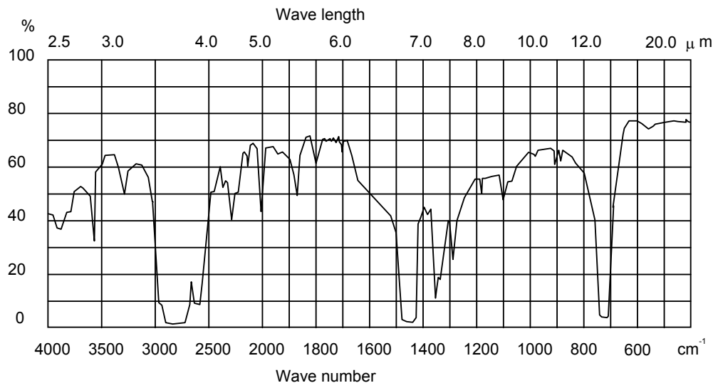
第 2 図 赤外分光透過特性 Figure 2 Transmittance
