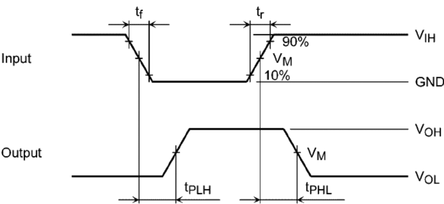
Fig. 9.7.1 t_{PLH} , t_{PHL}
