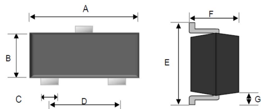
SOT-23
