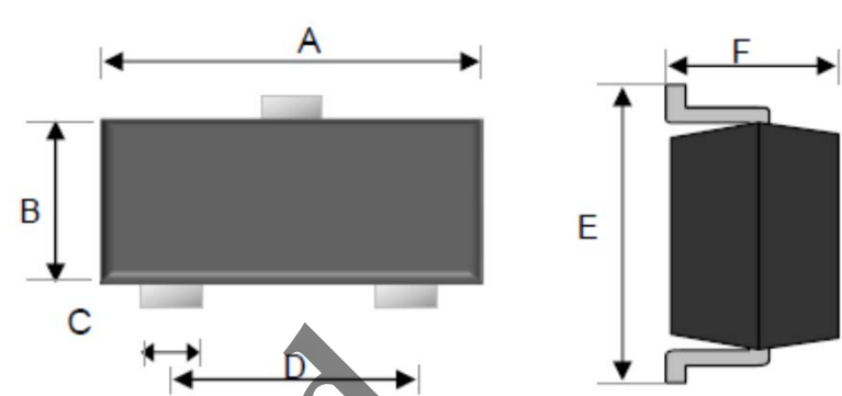
SOT-323
