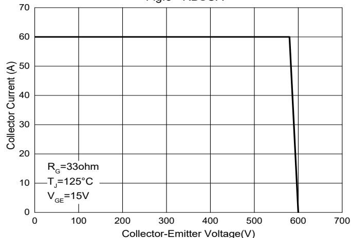
Fig.5 - RBSOA
