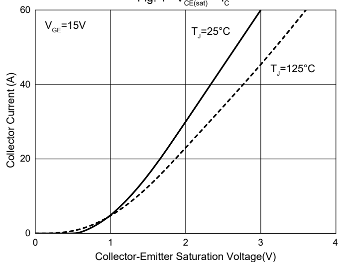
Fig. 1 - V_{CE(sat)} - I_C
