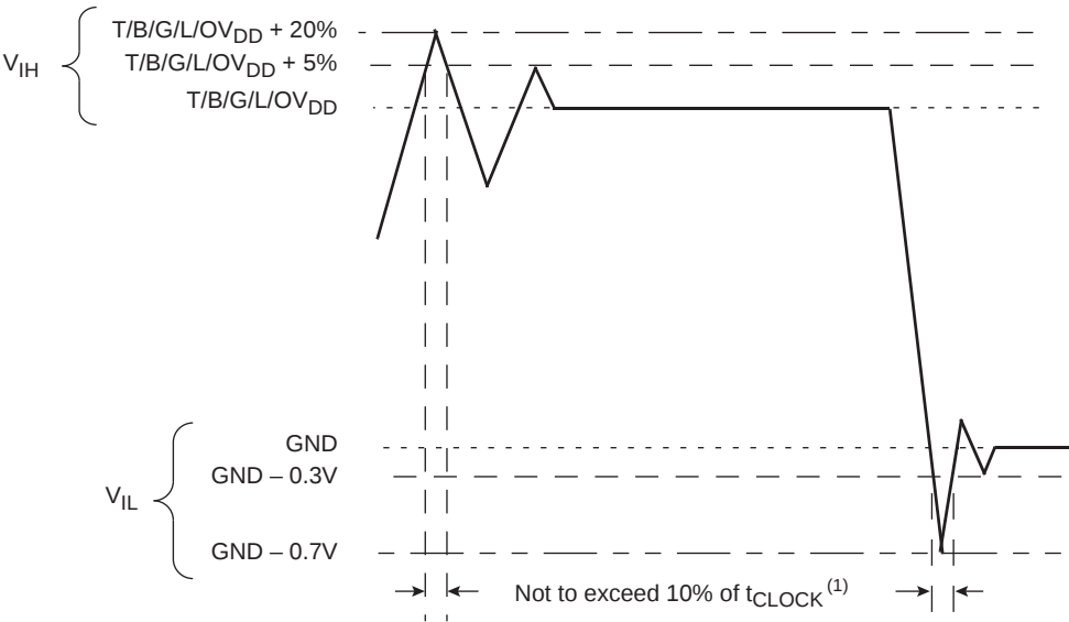
Figure 2-1. Overshoot/Undershoot Voltage for TV DD /BV DD /GV DD /LV DD /OV DD
