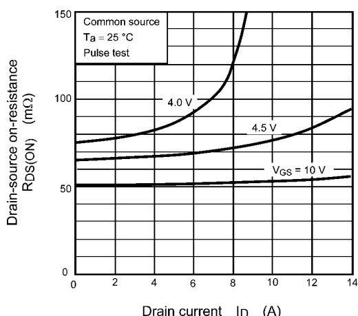
Fig. 9.4 R_{DS(ON)} - I_D
