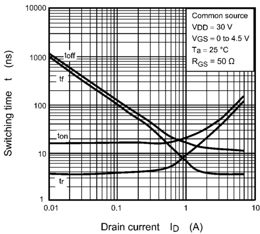
Fig. 9.9 t - I_D
