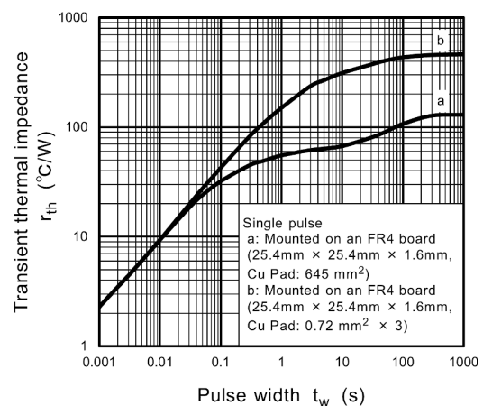
Fig. 9.12 r_{th} - t_w
