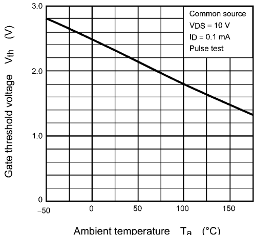
Fig. 9.6 V_{th} - T_a
