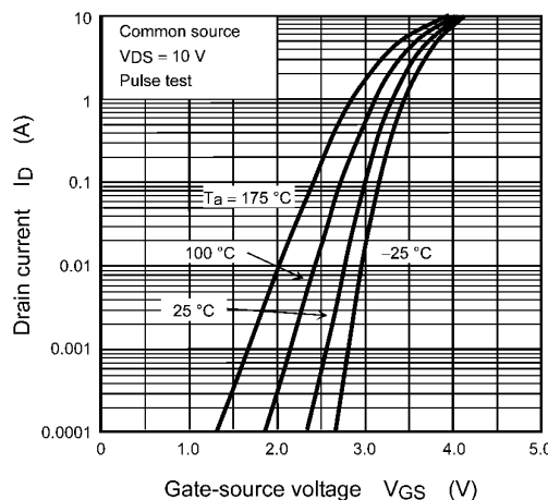
Fig. 9.2 I_D - V_{GS}
