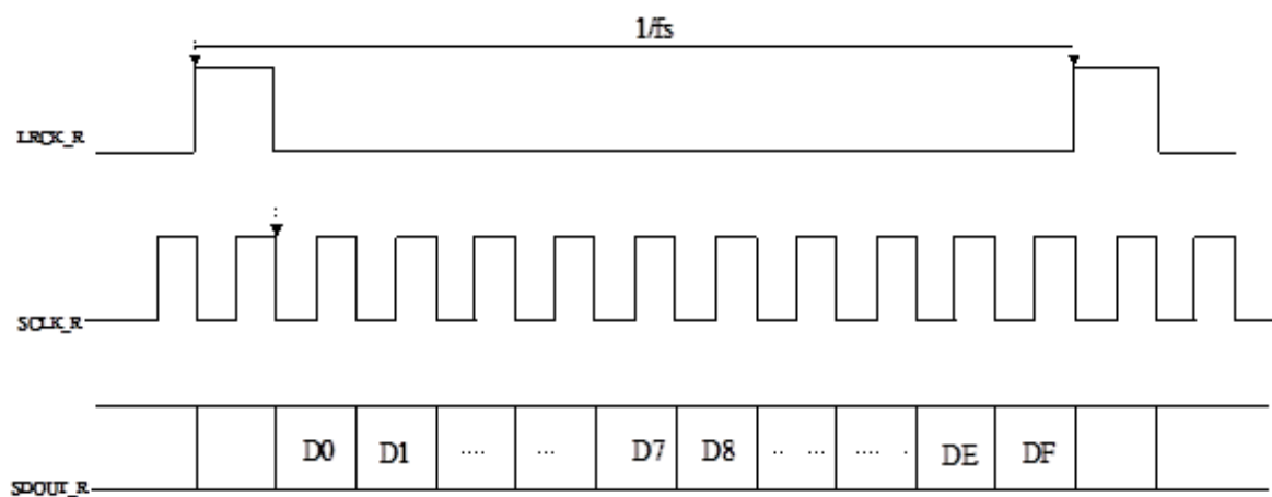
DSP mode
