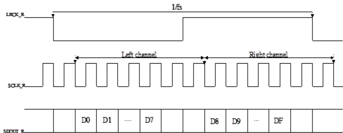
I2S mode
