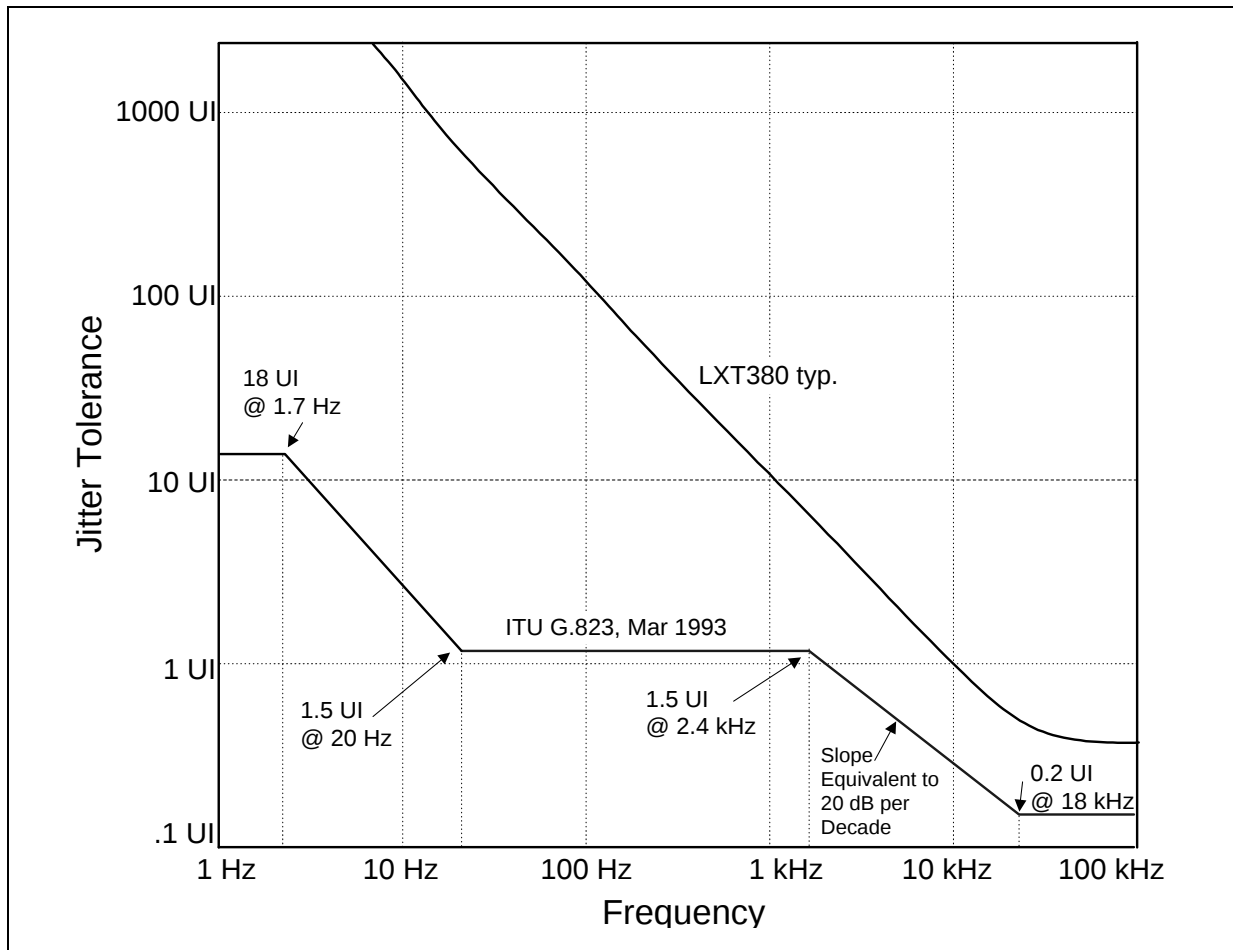
Figure 31. E1 Jitter Tolerance
