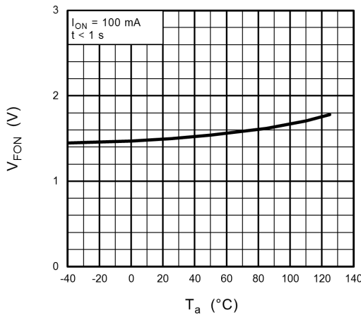
Fig. 12.5 V_{FON} - T_a
