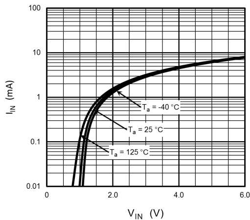
Fig. 12.1 I_{IN} - V_{IN}
