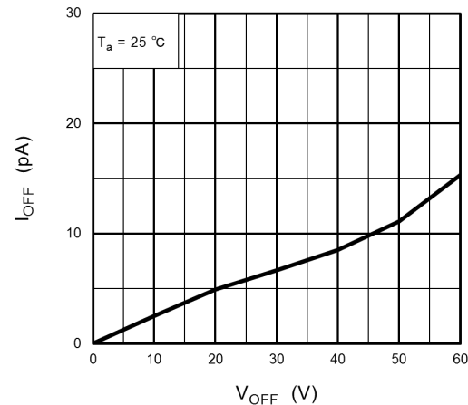
Fig. 12.8 I_{OFF} - V_{OFF}
