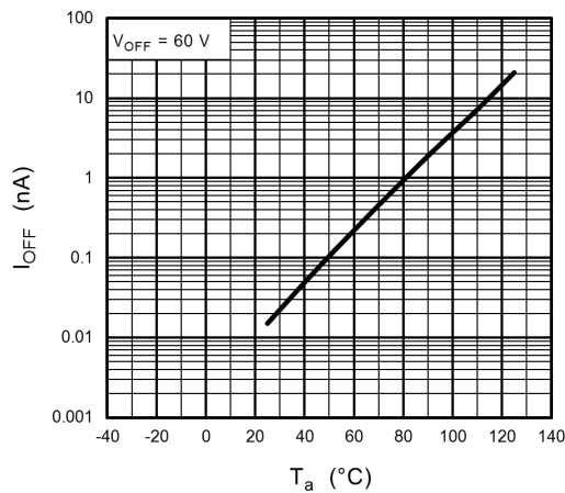
Fig. 12.9 I_{OFF} - T_a
