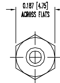
HEX NUT
