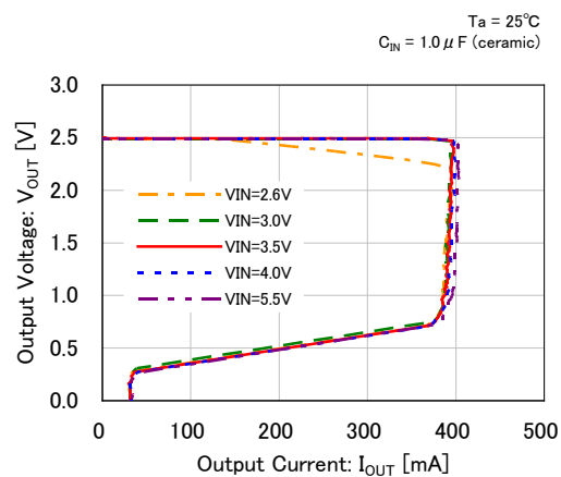
XC6229x251
