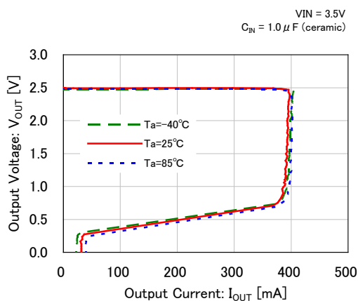
XC6229x251
