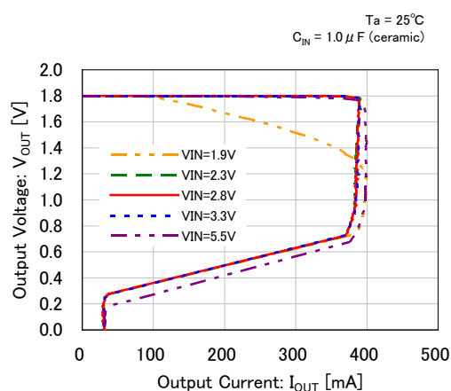
XC6229x181
