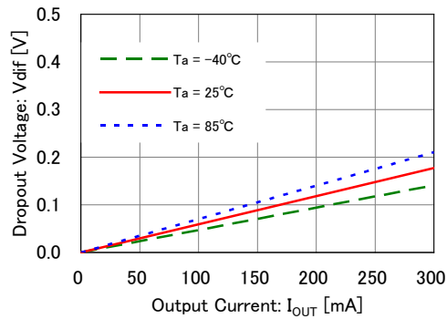
XC6229x251
