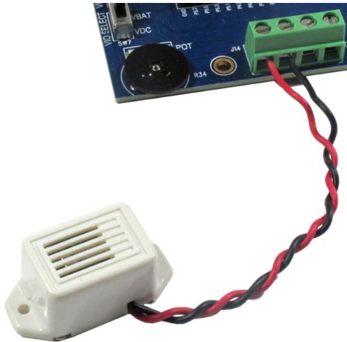
Figure 27. Optional 3 V Buzzer
