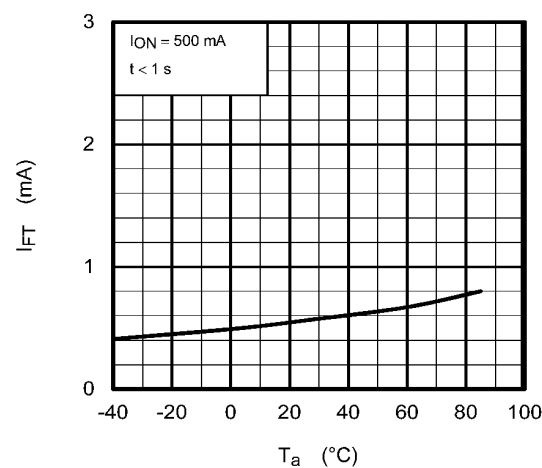
Fig. 14.6 I_{FT} - T_a
