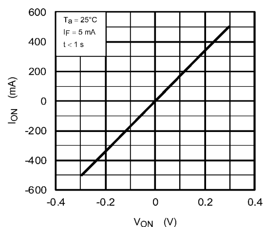
Fig. 14.4 I_{ON} - V_{ON}
