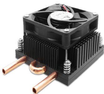
ATS-LQHS-84025-C1-R0 84.0 x 84.0 x 25.8mm Thermal Resistance: 0.05°C/W
