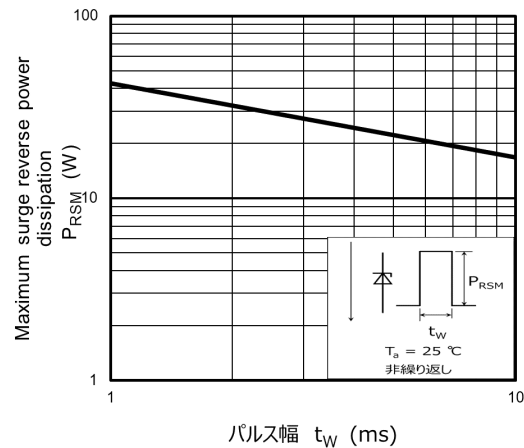
Fig. 10.1.2 P_{RSM} - t_W
