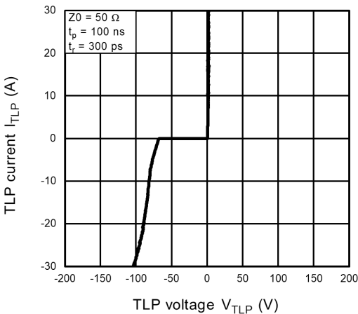
Fig. 10.4.1 I_{TLP} - V_{TLP}
