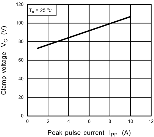
Fig. 10.4.2 V_C - I_{PP}
