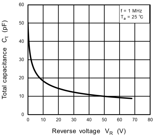
Fig. 10.4.3 C_T - V_R
