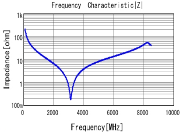
■ GCQ1555C1H7R4CB01 |Z| DC0V, 25degC
