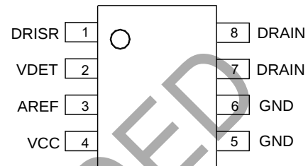
SO-8
