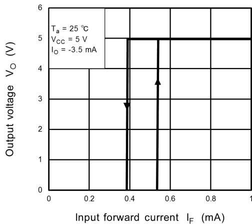
Fig. 13.2.3 V_O - I_F(I_{HYS})
