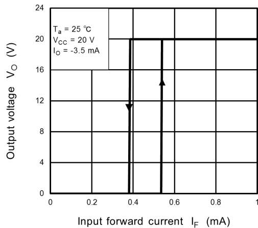
Fig. 13.2.4 V_O - I_F(I_{HYS})
