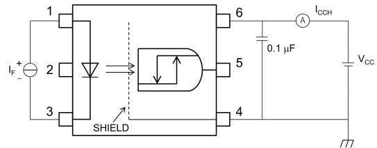
Fig. 13.1.4 I_{CCH} Test Circuit
