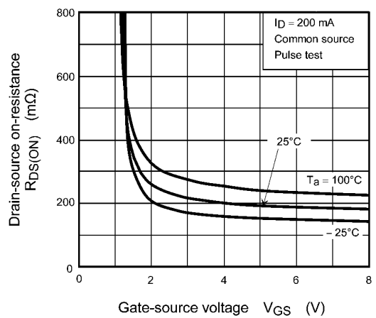
Fig. 7.3 RDS(ON) - VGS
