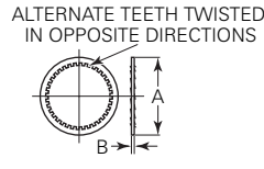
Lockwasher
