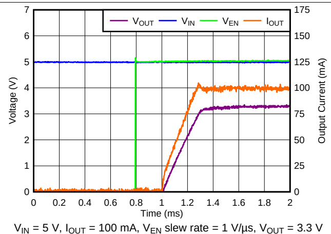
Figure 12. EN Startup
