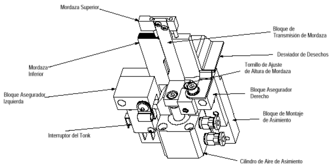
Subensamble de Asimiento
