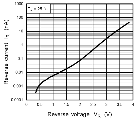
Fig. 7.2 I_R - V_R
