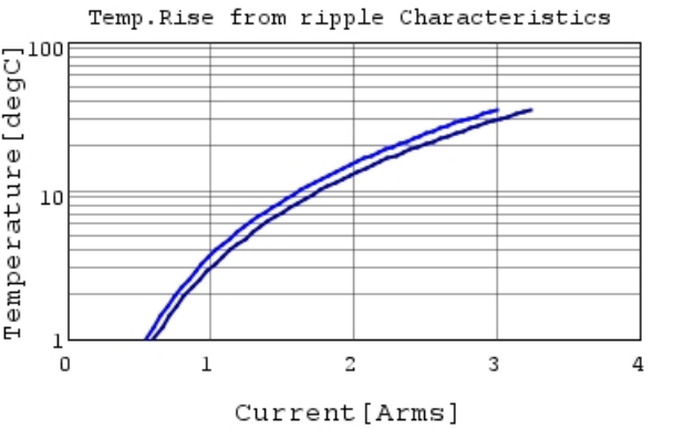
GRM033R60J225ME15 Temp.rise — 500kHz —
