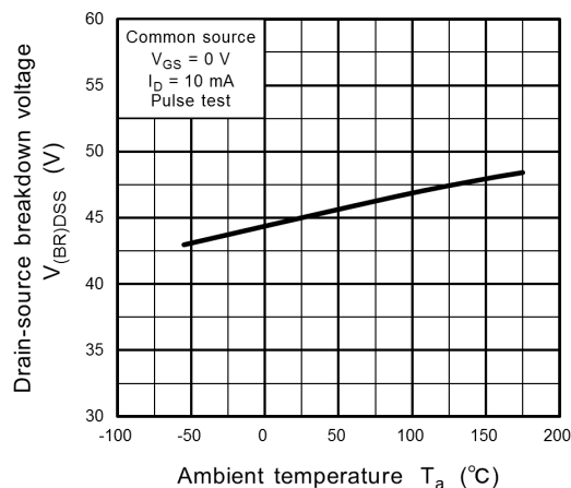
Fig. 8.11 V_{(BR)DSS} - T_a
