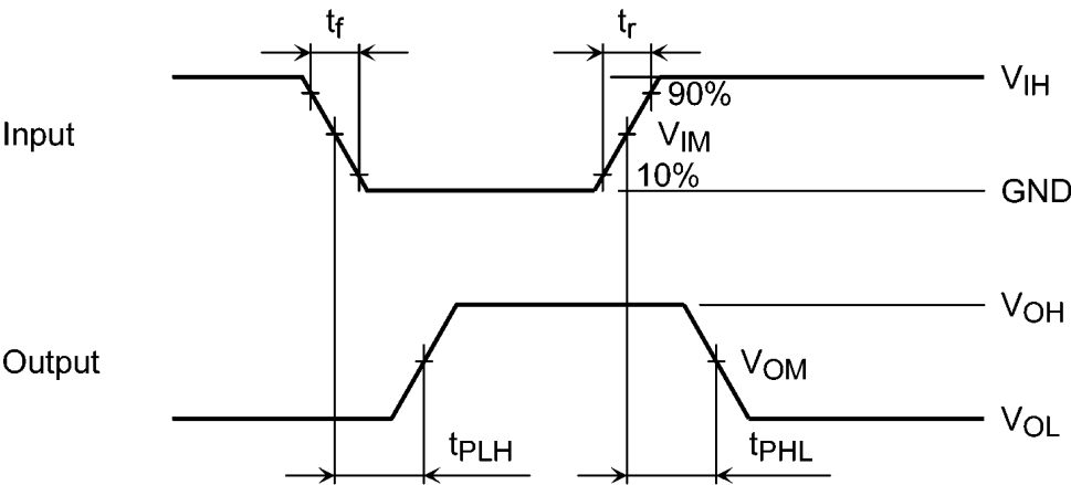
Fig. 11.8.1 t_{PLH}, t_{PHL}
