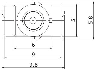
5.4 MM ACTUATOR
