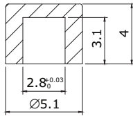
ACTUATOR CAP
