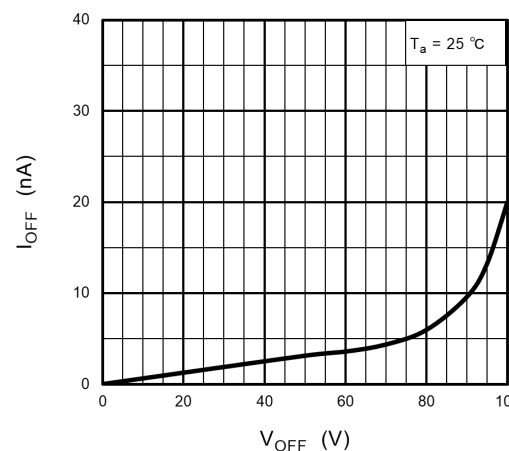
Fig. 12.1.10 I_{OFF} - V_{OFF}
