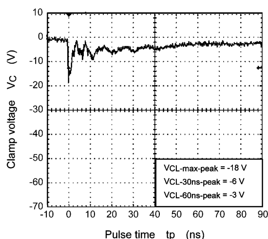
Fig. 9.2 -8 kV
