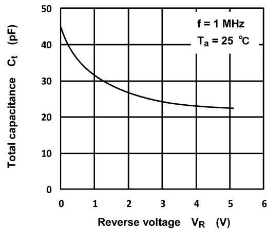
Fig. 7.3 C_t - V_R
