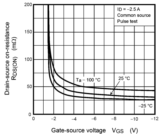
Fig. 9.4 R_{DS(ON)} - V_{GS}
