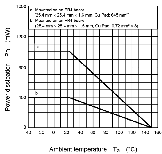
Fig. 9.14 P_D - T_a
