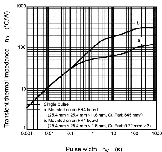
Fig. 9.13 r_{th} - t_w
