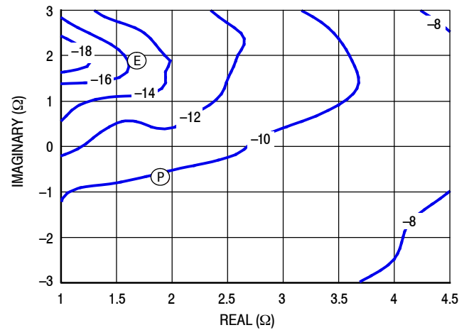
Figure 27. P1dB Load Pull AM/PM Contours (°)
