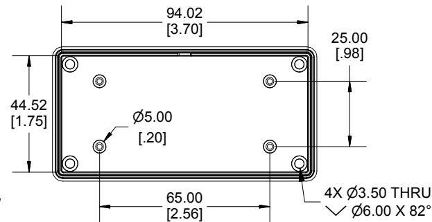
INSIDE LID
