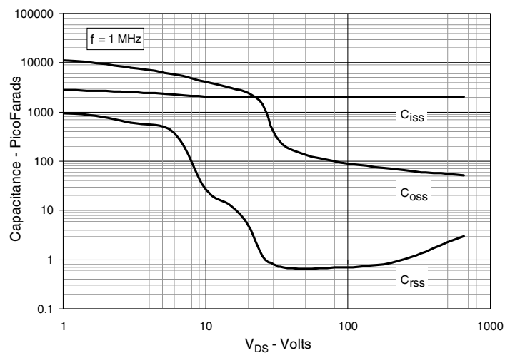
Fig. 12. Capacitance
