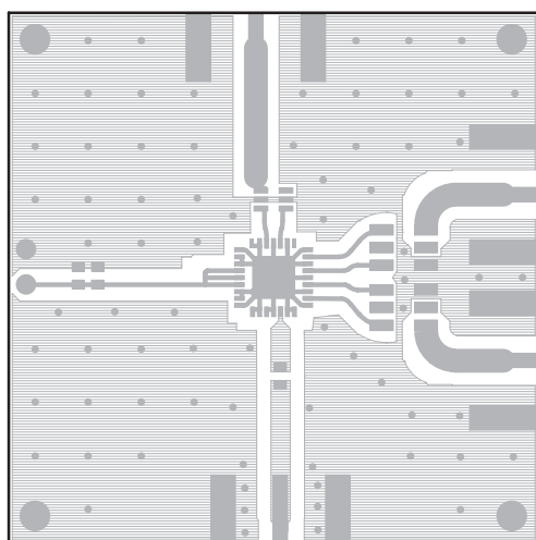
Top Layer
