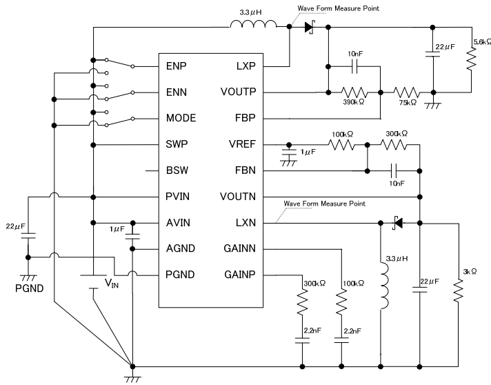
9) Circuit ⑨
