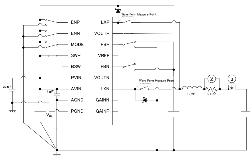
6) Circuit ⑥
