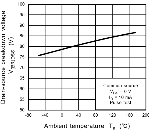
Fig. 8.7 V_{(BR)DSS} - T_a
