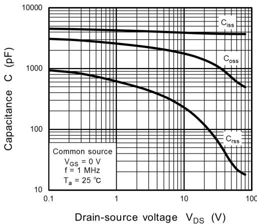
Fig. 8.11 Capacitance - V_{DS}
