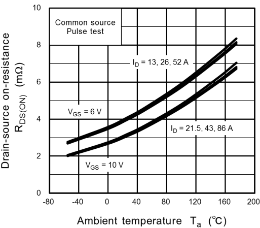
Fig. 8.9 R_{DS(ON)} - T_a
