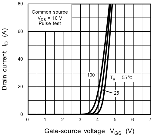
Fig. 8.3 I_D - V_{GS}
