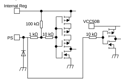
3) PS pin
