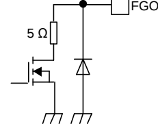
12) FGO pin
