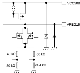
5) FR pin
